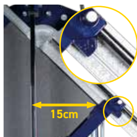
Dubbele maataanduiding
